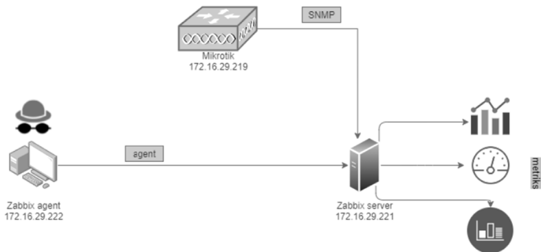
Рис. 1. Проектировка стенда
