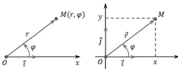
Рис. 1. Построение точки в полярной системе координат
