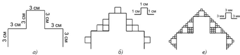
Построение геометрического фрактала: а) шаг первый; б) шаг второй; в) шаг третий
