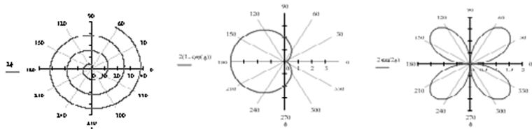
Рис. 2. Графики в полярной системе координат
