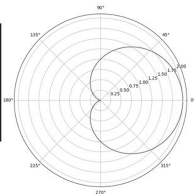
Рис. 6. Кардиоида
