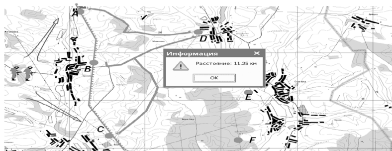
Рис. 2. Возможные маршруты от позиции D к пунктам A, B, C
